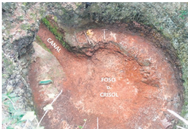
◻ Izq.: Uno de los hornos analizados en Azarola, Usansolo. Dcha.: Estructura de los hornos.
